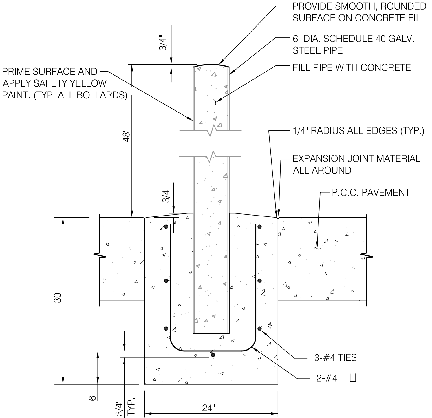
0502 BOLLARD - EMBEDDED SCALE: NTS
