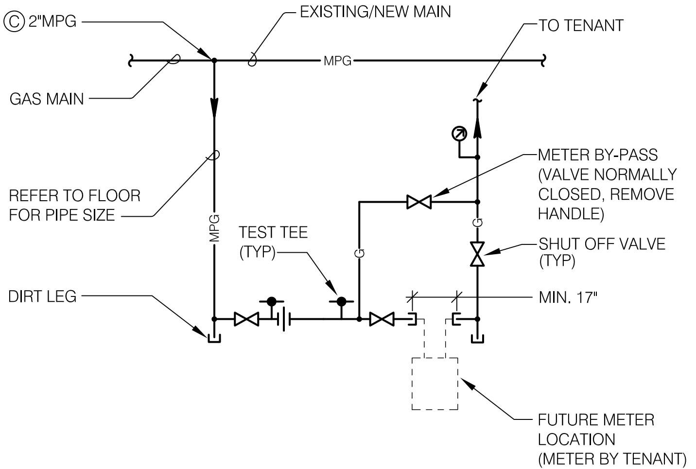
2201 GAS METER 1 SCALE: NTS
